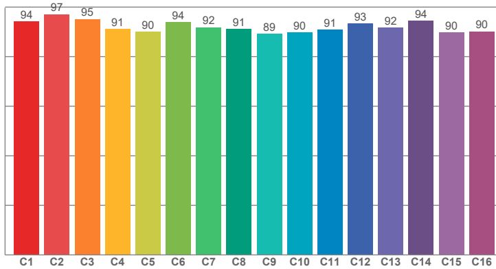
TM30: 92,0
