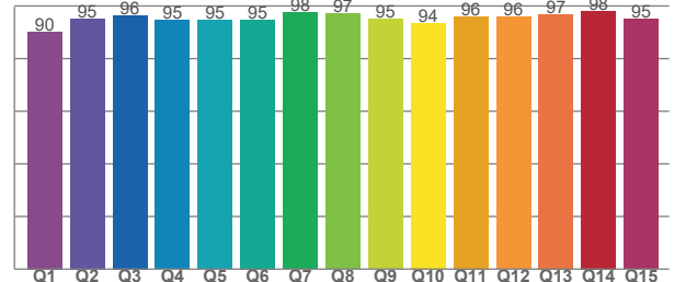
CQS: 95,1
